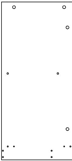
2 ( 15 x 363 x 795 mm ) ( 0,59 x 14,29 x 31,30 in )
